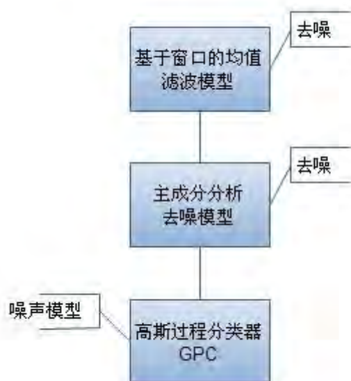
图 5.3.1 去噪模型
