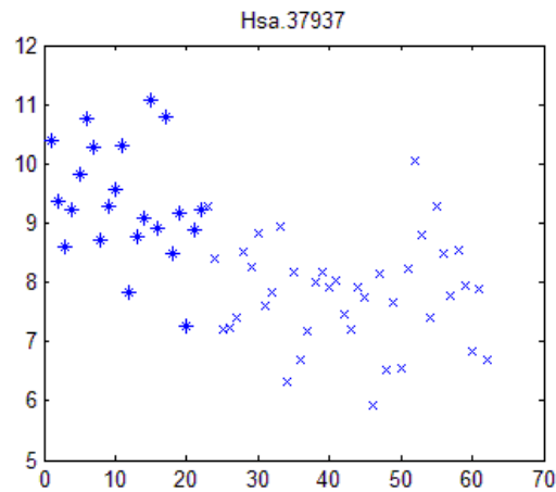
图5.2.3 基因标签Has.37937在不同样本的表达水平
