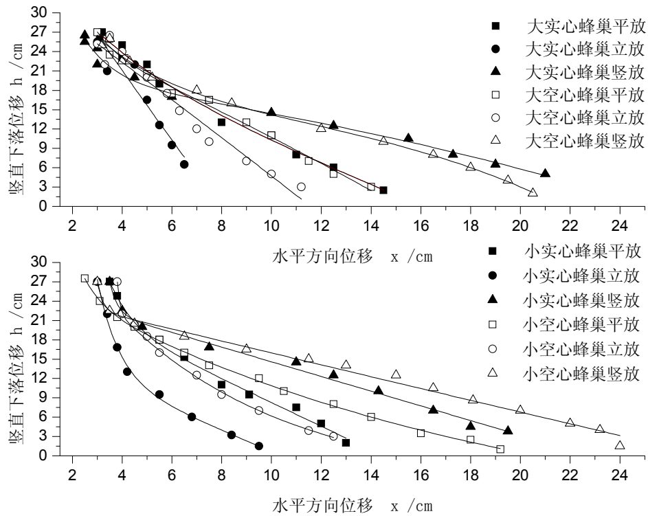
附图 2.4 蜂巢 5cm 下落, 0.40m/s 时的运动轨迹
