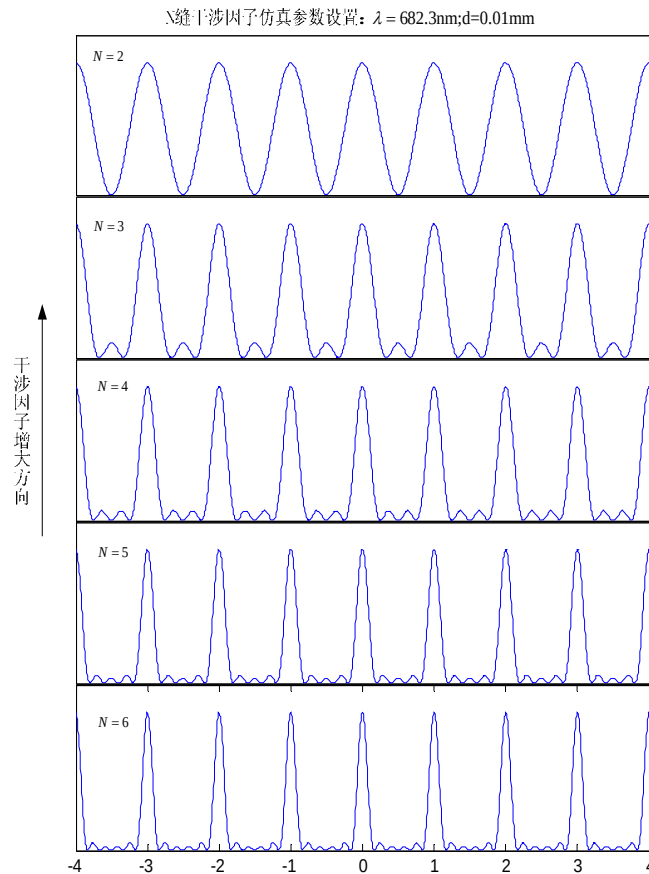
图 5.2 缝间干涉因子曲线
