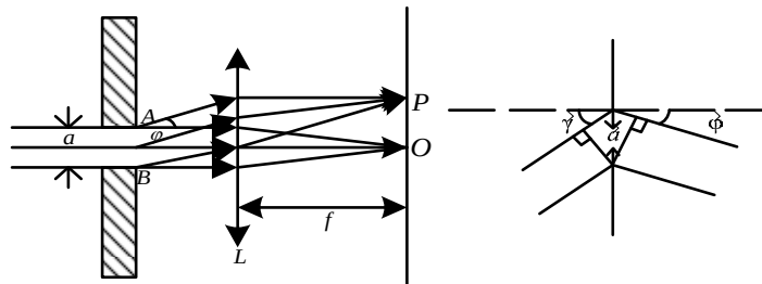
图 3.1 单缝衍射的示意图
