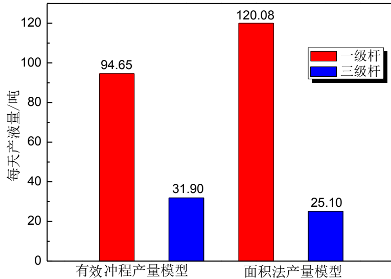
图 3-9 不同产量模型预测油井产量对比图
