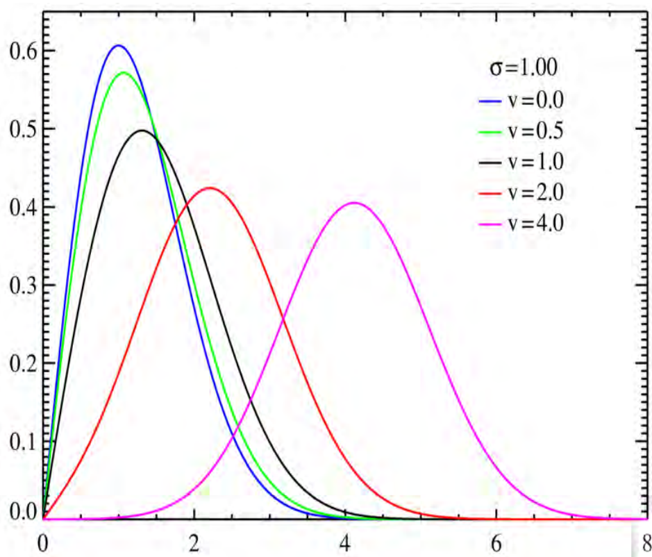
图 7.6 莱斯分布图
