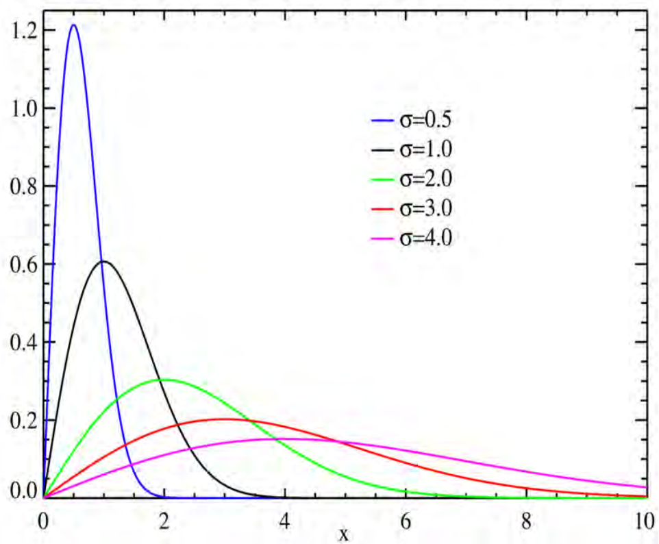
图 7.5 瑞利分布图
