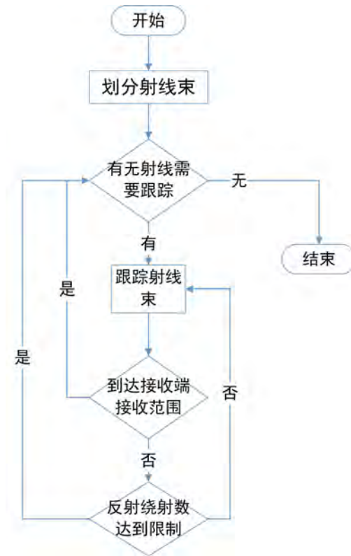
图 13: 量化射线追踪法算法流程图。
