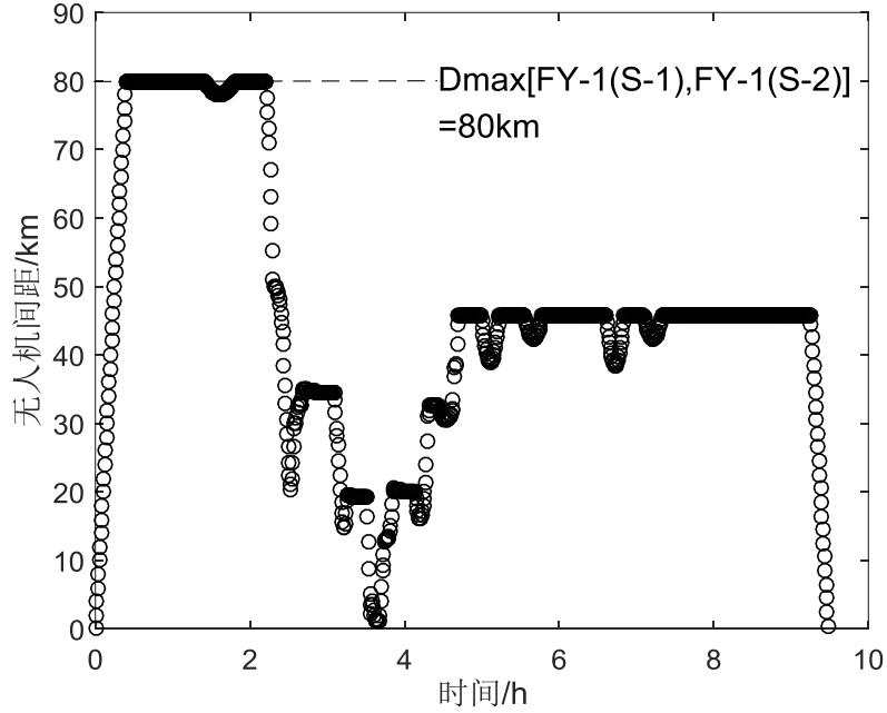
图 15 t_l=0.2h ，P1 基地起飞的两无人机间距随时间变化
