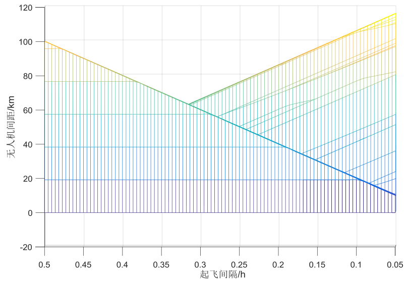
图 17 P1 基地起飞的无人机最大间距与起飞间隔的关系 据此调整： t_I=0.38h ，使得两架无人机之间最大距离为 65km。
