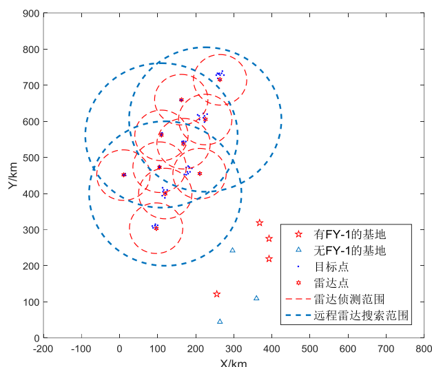
图 29 远程雷达探测范围
