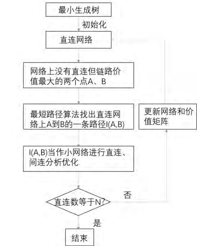
图 10 算法流程图
