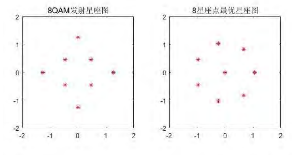
图 20 8QAM 星座图与 8 点最佳星座图对比
