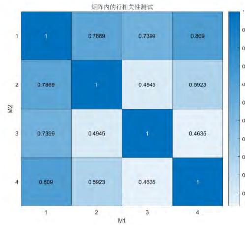
图 6 j = 1, k = 10 矩阵内的行相关系数
